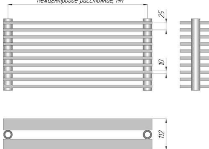
Параллели Г2 шаг 25
