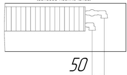
Конвектор Бриз (боковое подключение)
