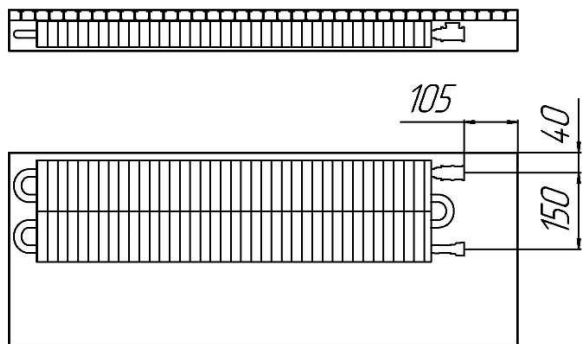
Расположение теплообменников в конвекторах Бриз шириной 380 (сечение)
