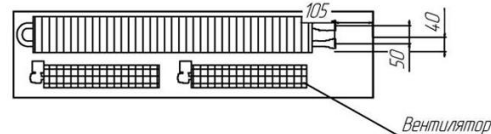
Конвектор Бриз В шириной 360 (вид сверху)
