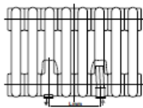
рис. 1 L=45 x (кол-во секций между двумя муфтами (секции с сварными муфтами) – 1)
