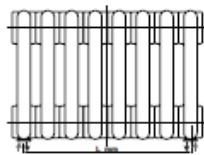
рис. 2 L=45 x (кол-во секций в батарее – 1)
